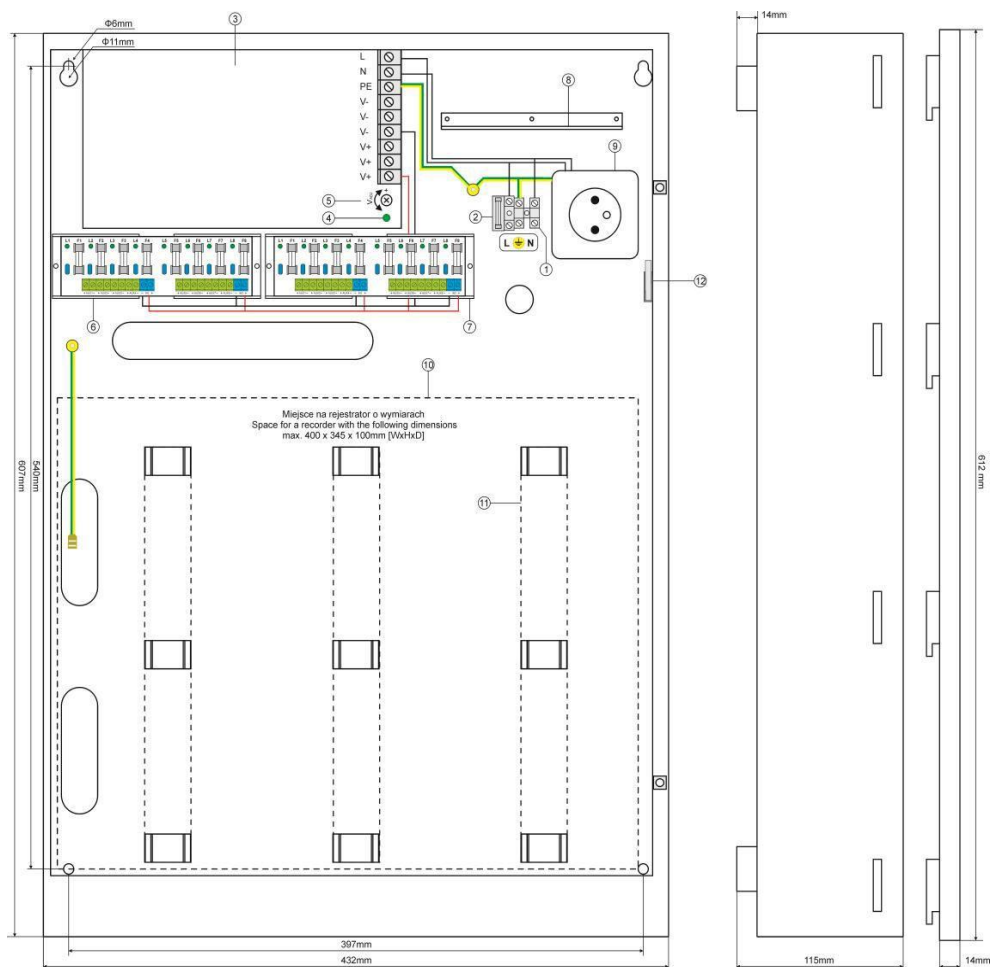
Obr.3. Náhled napájecího zdroje.
