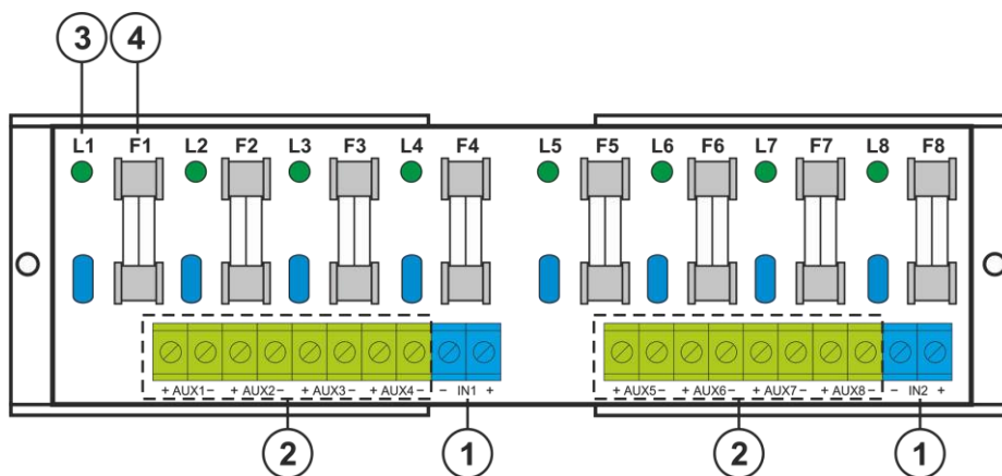
Obr. 2. Náhled na pcb jedné desky (ze dvou).
